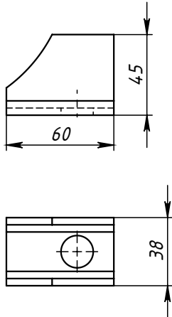
Поз.4 (Ушко)
