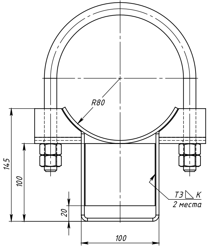
Поз.3 (Ложемент)
