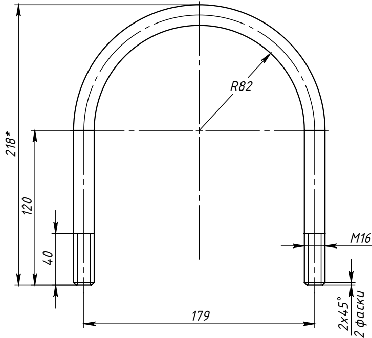
Поз.5 (Хомут)
