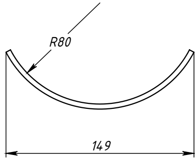
Поз.5 (Хомут)
